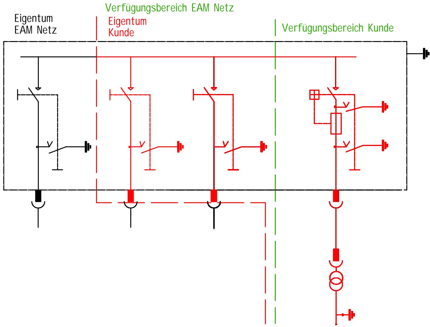
Prinzipschaltbild
