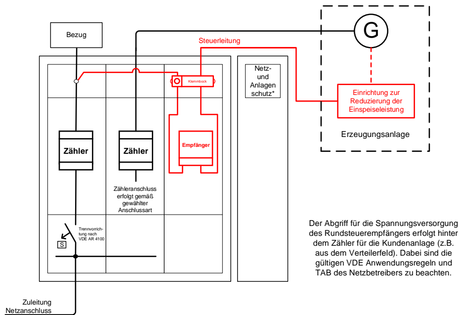
Abbildung 3 Einbindung der Empfängereinrichtung und Klemmbock bei einer Photovoltaikanlage am zentralen Zählerplatz in der Standardbauweise bei Installation eines Rundsteuerempfängers
