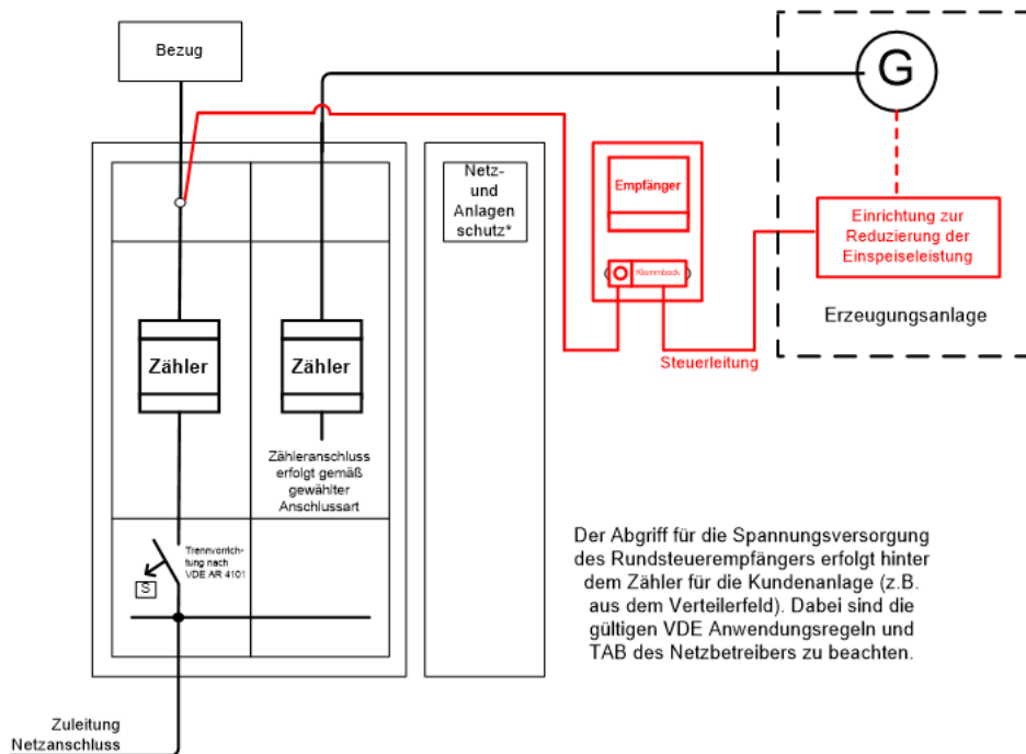
Abbildung 4 Einbindung der Empfängereinrichtung und Klemmbock bei einer Photovoltaikanlage am zentralen Zählerplatz in der Mindestbauweise bei Installation eines Rundsteuerempfängers
